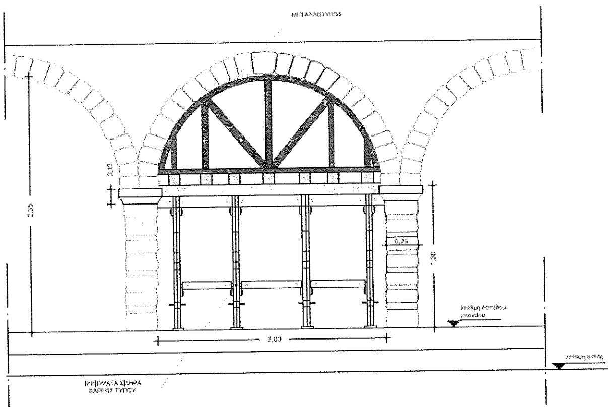
ΛΕΠΤΟΜΕΡΕΙΕΣ ΥΠΟΣΤΥΛΩΣΗΣ ΤΟΞΟΣΤΟΙΧΕΙΑΣ
